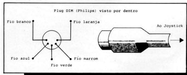
Figura 3 — Ligação dos fios do joystick.
